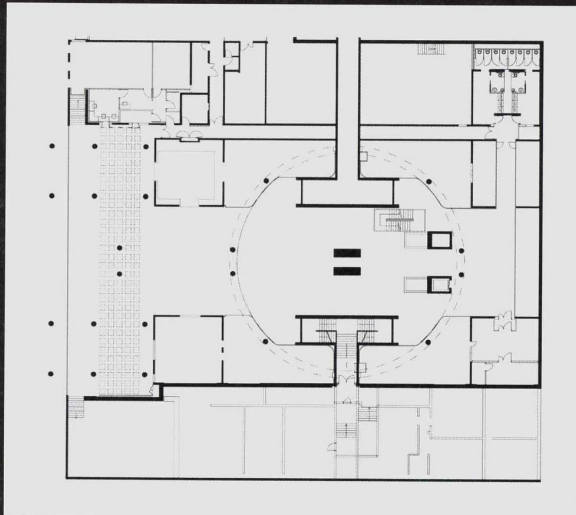
Plan du niveau 3 – rez-de-chaussée
